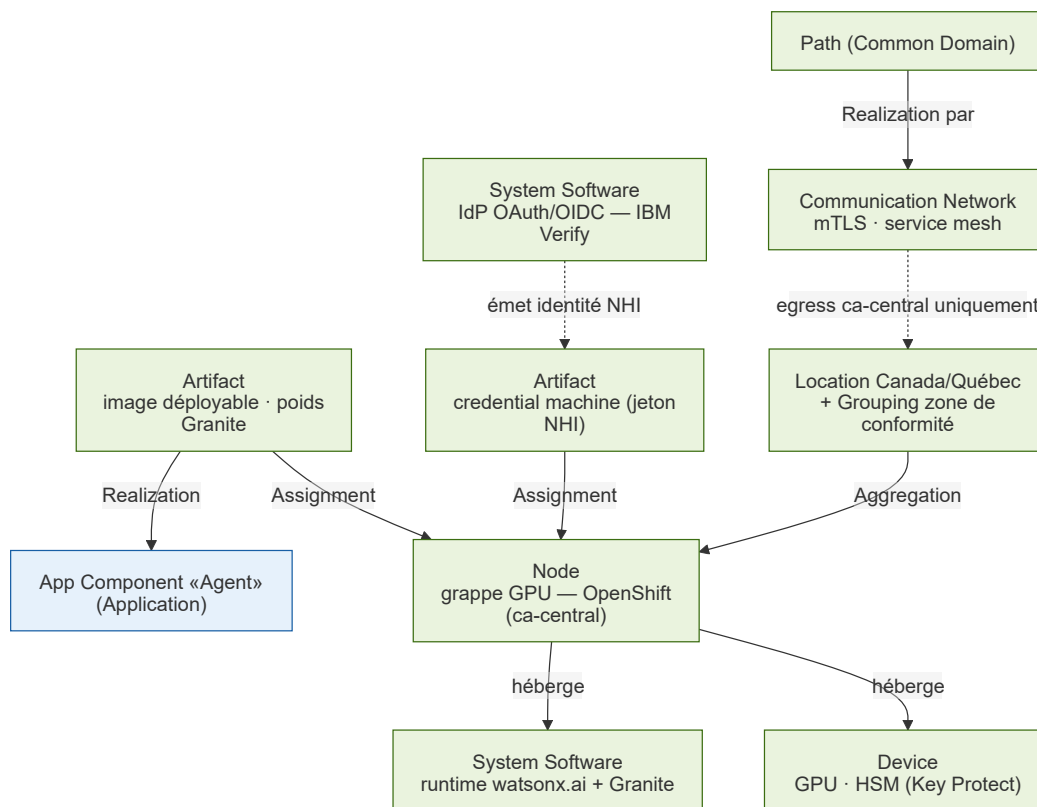
Figure G — Vue Technologie. Le substrat d'exécution confiné : l'Artifact (image, poids Granite) réalise l'Application Component et est assigné à un Node (grappe GPU OpenShift en ca-central) hébergeant le System Software (runtime) et les Device (GPU, HSM). Le credential machine (jeton NHI) est un Artifact assigné au Node ; le Path (Common Domain v4) est réalisé par un Communication Network (mTLS) ; la Location et le Grouping de zone fixent la résidence — l'absence de Path sortant traduisant l'interdiction d'egress.
